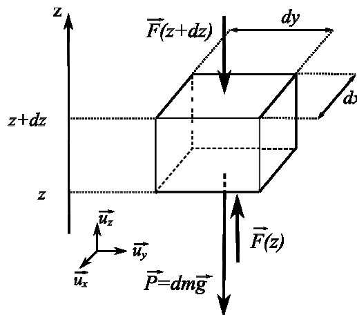
Figure I.6. Volume élémentaire de fluide de forme cubique. Les arêtes du cube sont colinéaires à un système d'axes orthogonaux Oxyz . \vec{F}(z) et \vec{F}(z + dz) représentent les vecteurs forces de pression sur les deux faces du cube perpendiculaires à Oz et situées respectivement en z et z + dz .
