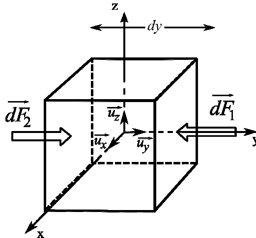
Figure I.7. Volume élémentaire de fluide de forme cubique. Les arêtes du cube sont colinéaires à Ox, Oy ou Oz. d\vec{F}_1 et d\vec{F}_2 représentent les vecteurs forces de pression sur les deux faces du cube perpendiculaires à Oy et situées respectivement en y = dy/2 et y = -dy/2 .
