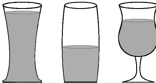
Figure I.1. Exemples de récipient de différentes formes – le contenu fluide adopte la forme du contenant.
