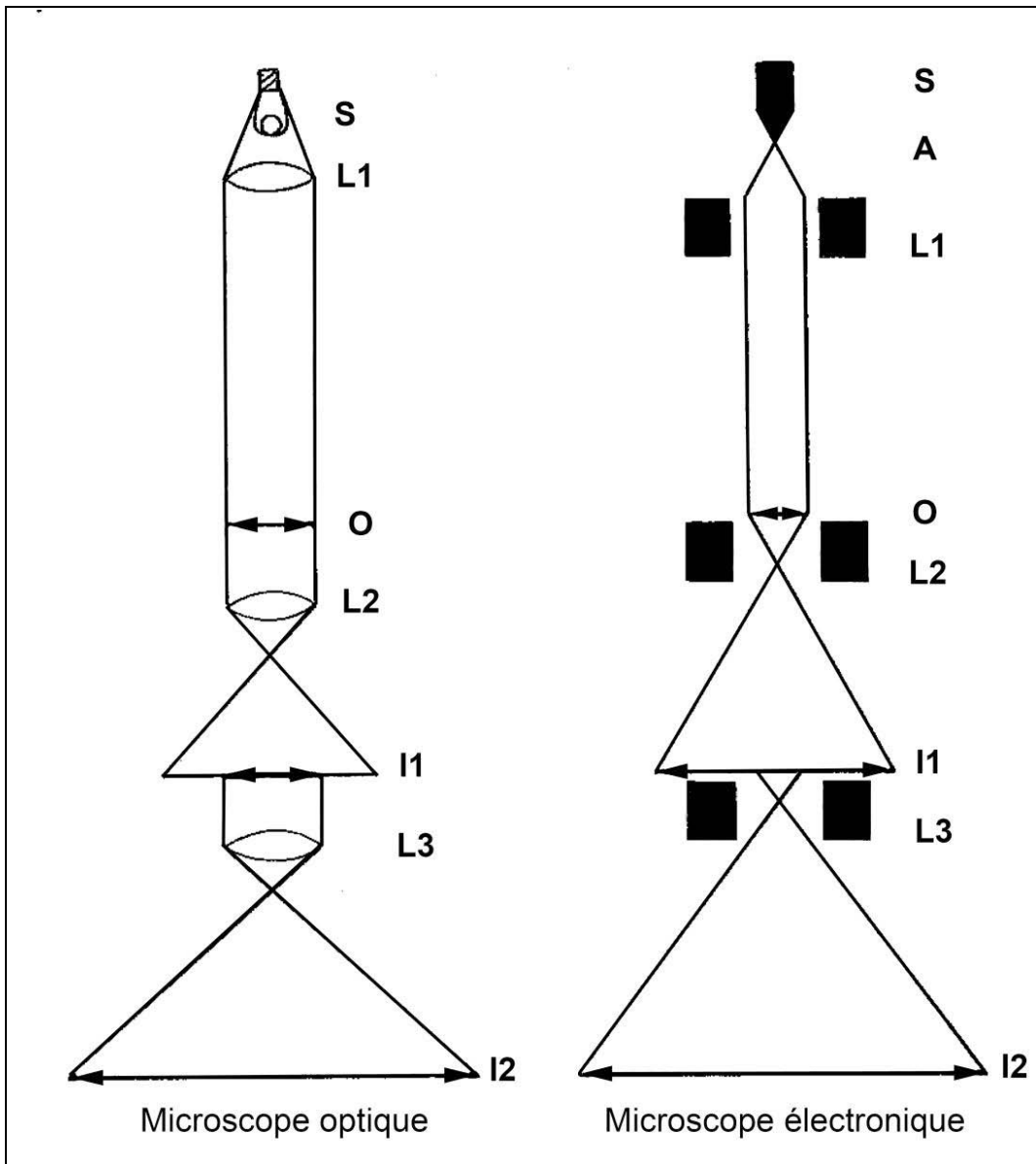
Figure 1. Principe du microscope optique et du microscope électronique (cf. texte).
