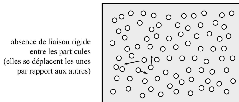
Figure 2.2 Disposition des particules à l'état liquide
