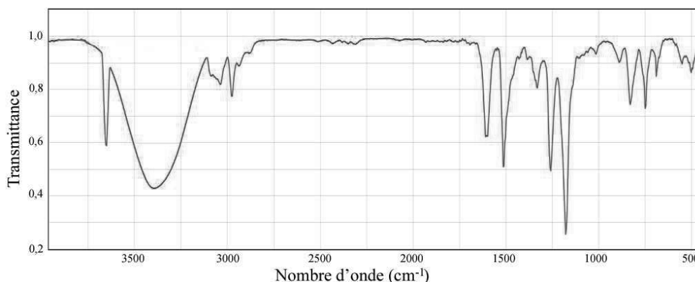
Figure 6b : Spectre d'absorption infrarouge du bisphénol A
