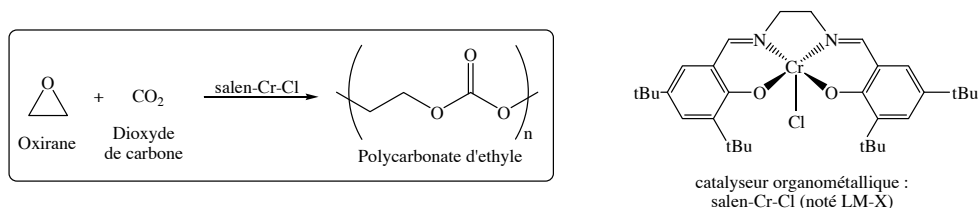
Figure 7 : Synthèse d'un polycarbonate par copolymérisation époxyde- \text{CO}_2
