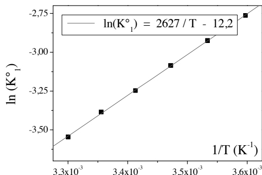
Figure 2 : Variation de K^{\circ}_1 avec la température
