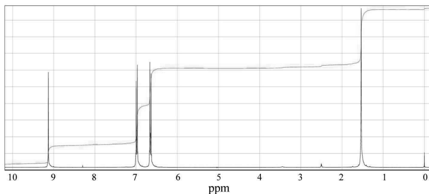
Figure 6a : Spectre RMN 1 H du bisphénol A
